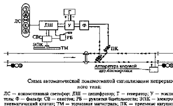
Рисунок 1 – Устройства АЛСН на станции
