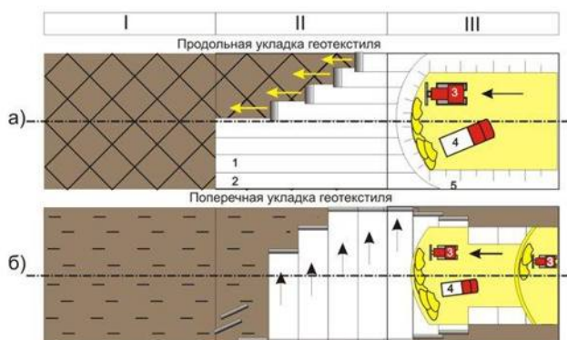
Рисунок 1 – Укладка геотекстиля
