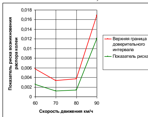
Зависимость показателя риска возникновения распада колеи от скорости движения
