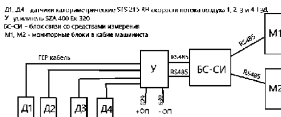
Рисунок 2 – Блок-схема системы оценки параметров охлаждения тяговых двигателей секции электровоза
